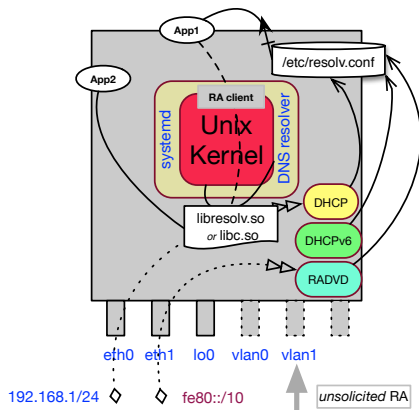
Abbildung: Nutzung und Management der Inhalte von /etc/resolv.conf
